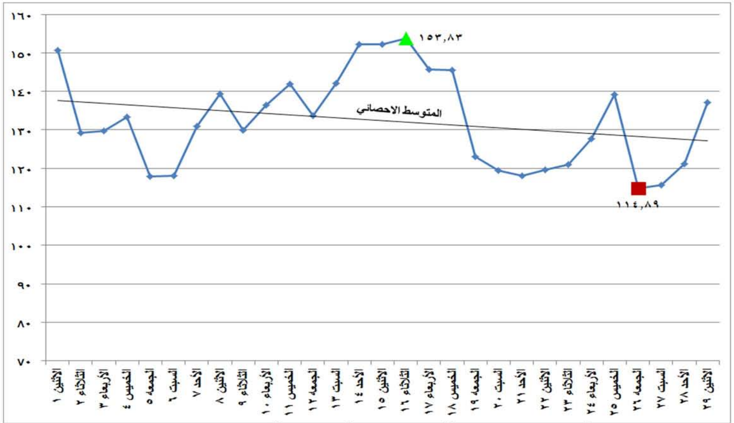
شكل (١٩) الطاقة الكهربائية المنتجة من المازوت خلال شهر فبراير ٢٠١٦
