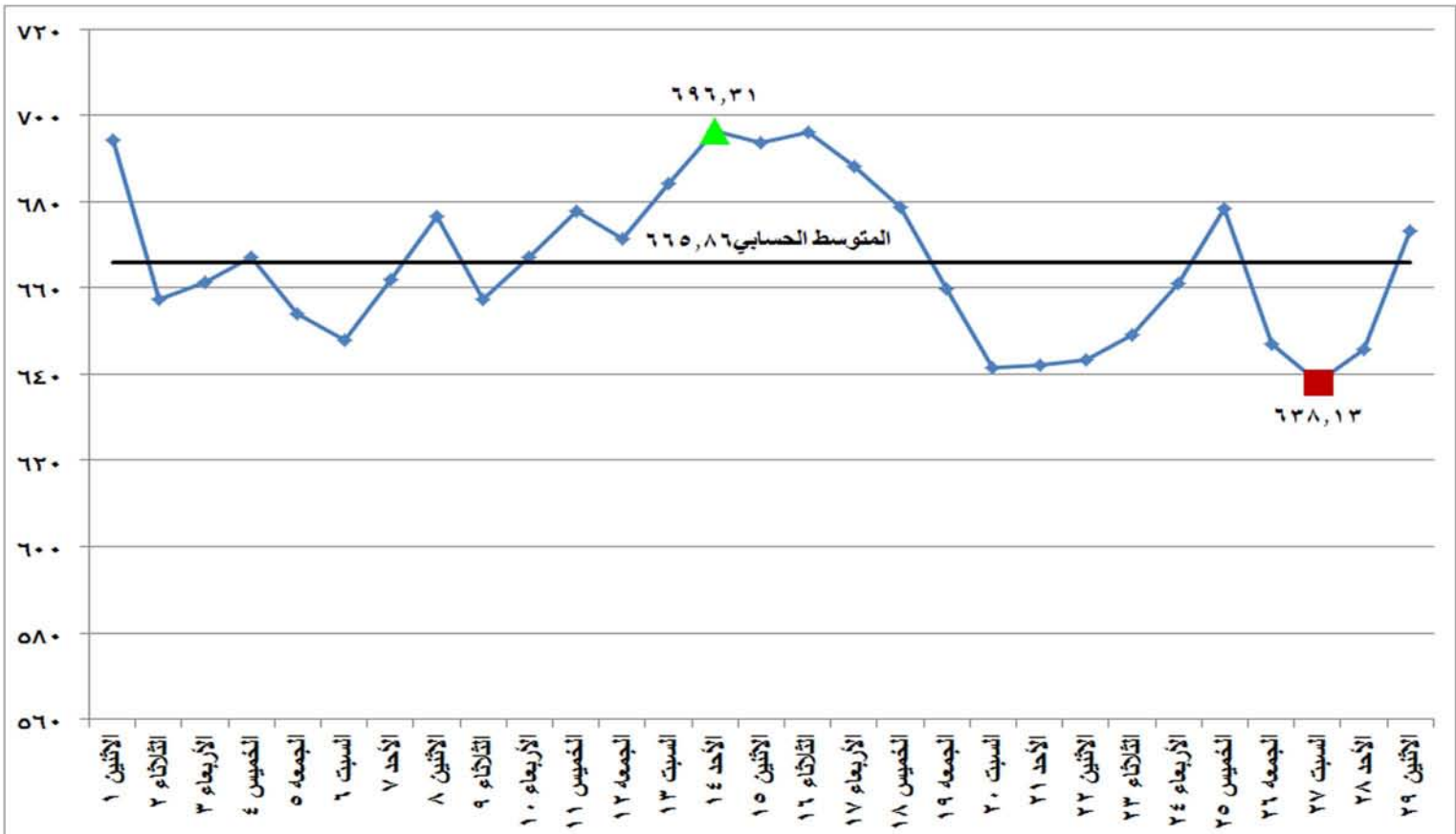
شكل (١٤) معامل انبعاثات غاز ثاني اكسيد الكربون المكافئ على مدى شهر فبراير ٢٠١٦
