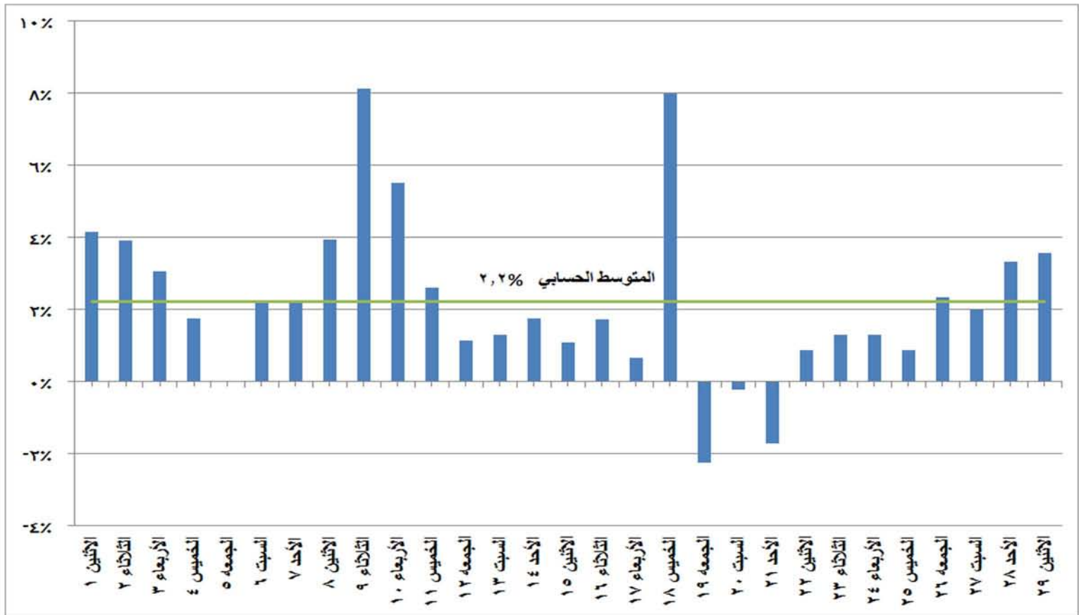
شكل (٩) النسب المئوية للتغير في الحمل الأقصى خلال شهر فبراير ٢٠١٦ مقارنة باليوم المماثل من العام الماضي
