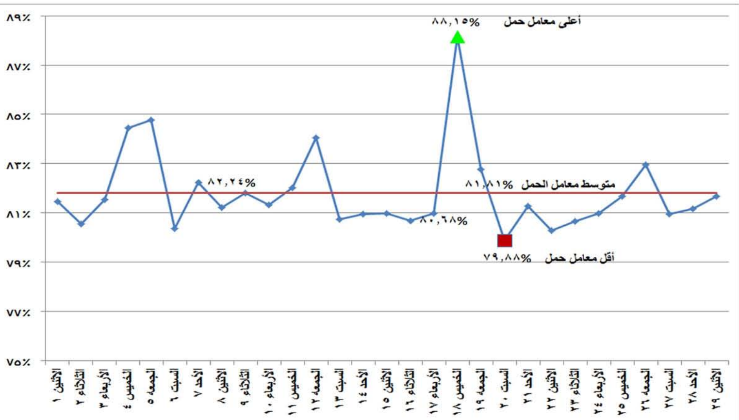
شكل (١٢) إجمالي معامل الحمل لوحدات الانتاج خلال شهر فبراير ٢٠١٦
