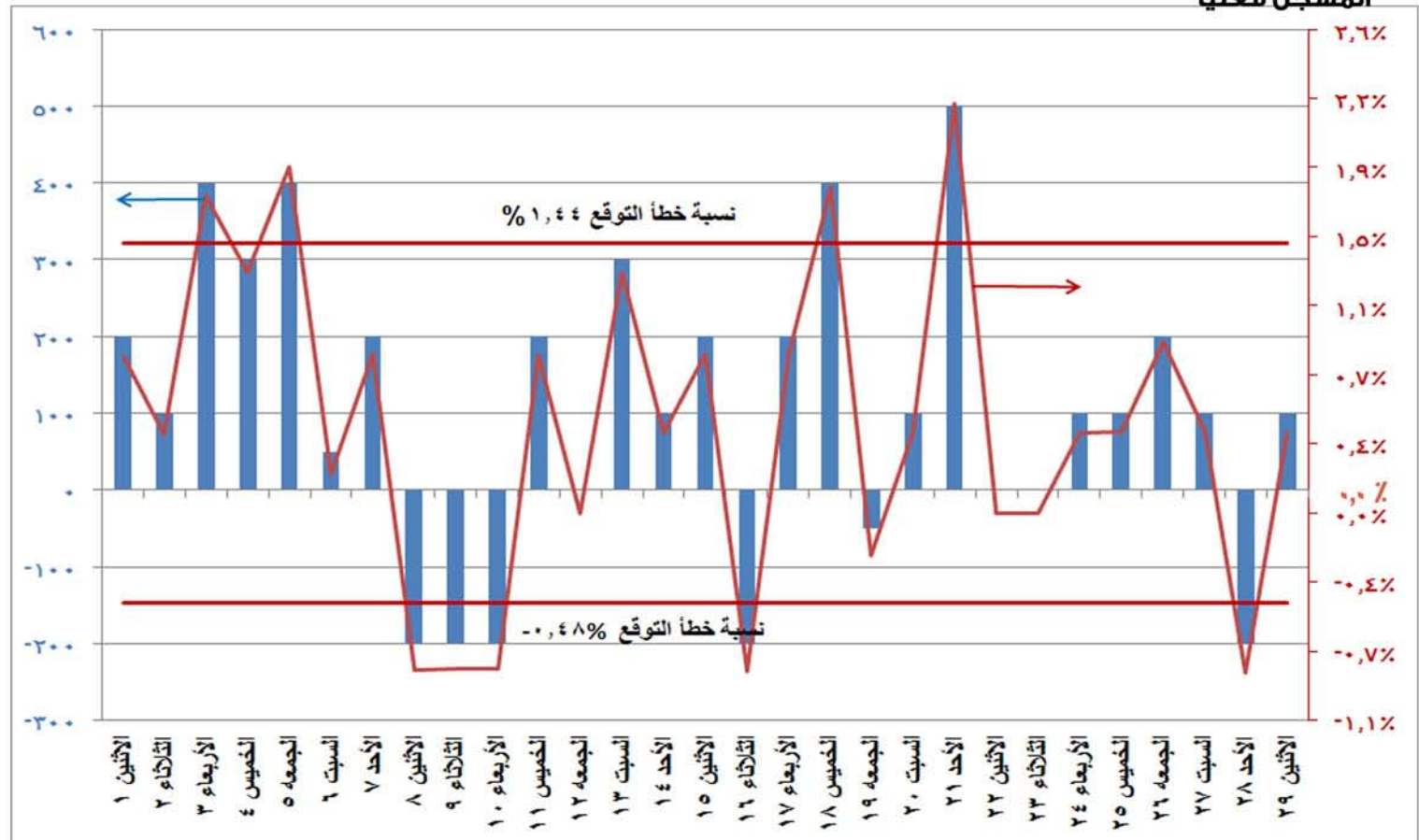
شكل (١٠) الفرق بين الحمل الأقصى المتوقع والحمل المسجل فعلياً ونسبة الفرق إلى الحمل المسجل فعلياً خلال شهر فبراير ٢٠١٦
