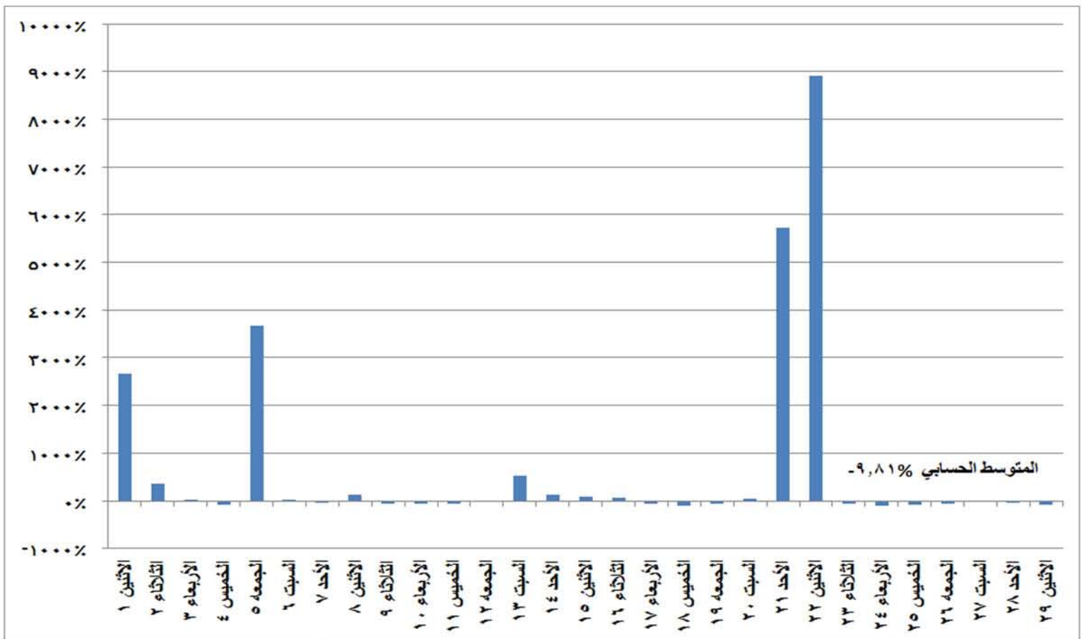
شكل (٢٦) نسب التغير في استخدام الرياح والشمس في إنتاج الطاقة الكهربائية خلال شهر فبراير ٢٠١٦ مقارنة بالشهر المماثل من العام السابق
