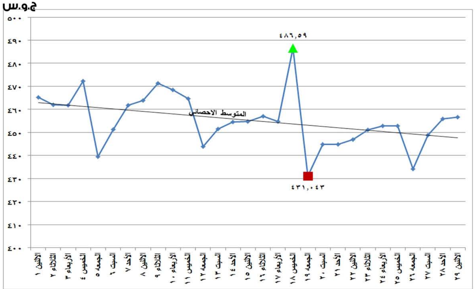
شكل (١٥) إجمالي الطاقة الكهربائية المنتجة من كل المصادر الأولية خلال شهر فبراير ٢٠١٦
