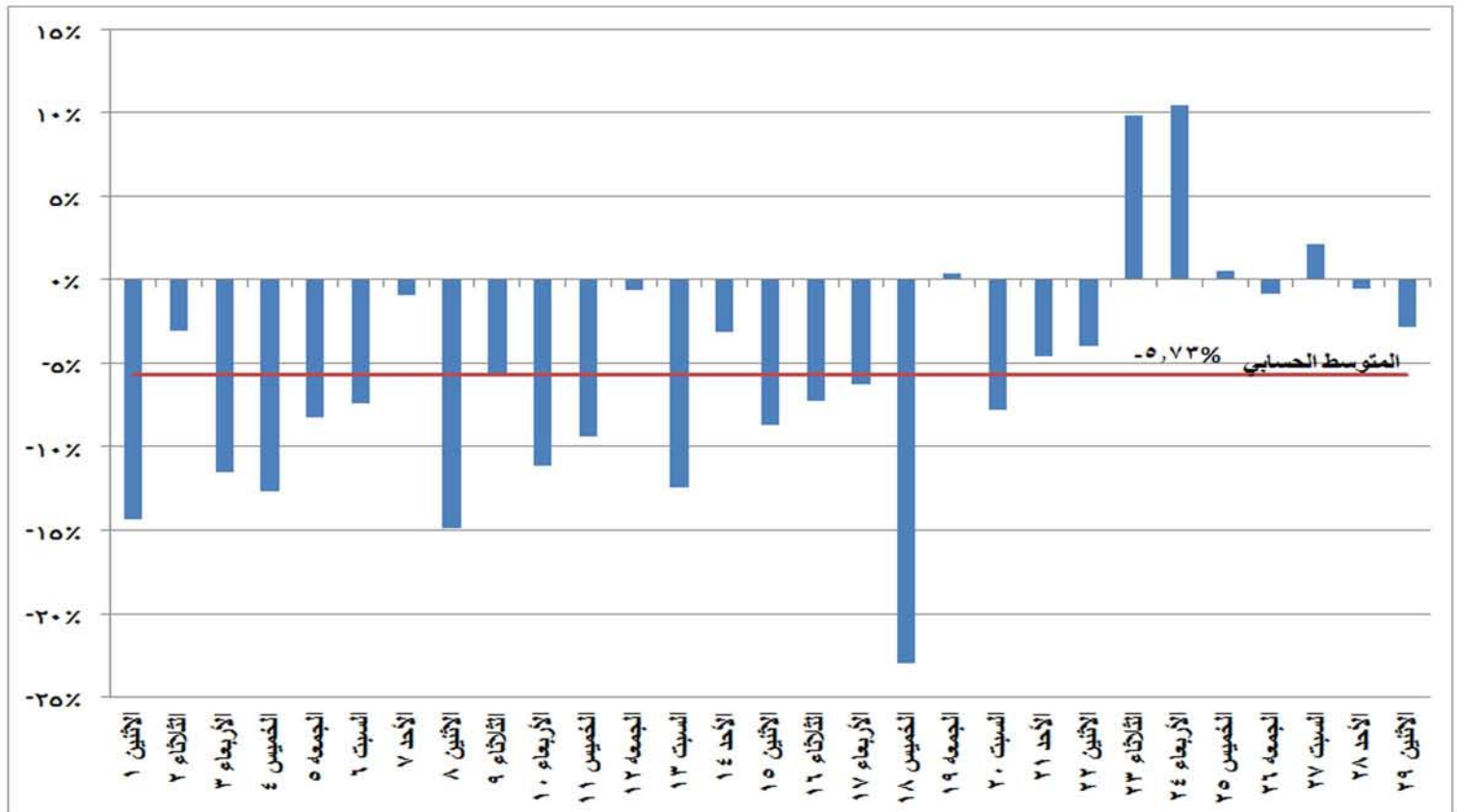
شكل (٢٤) نسب التغير في استخدام المصادر المائية في إنتاج الطاقة الكهربائية خلال شهر فبراير ٢٠١٦ مقارنة بالشهر المماثل من العام السابق
