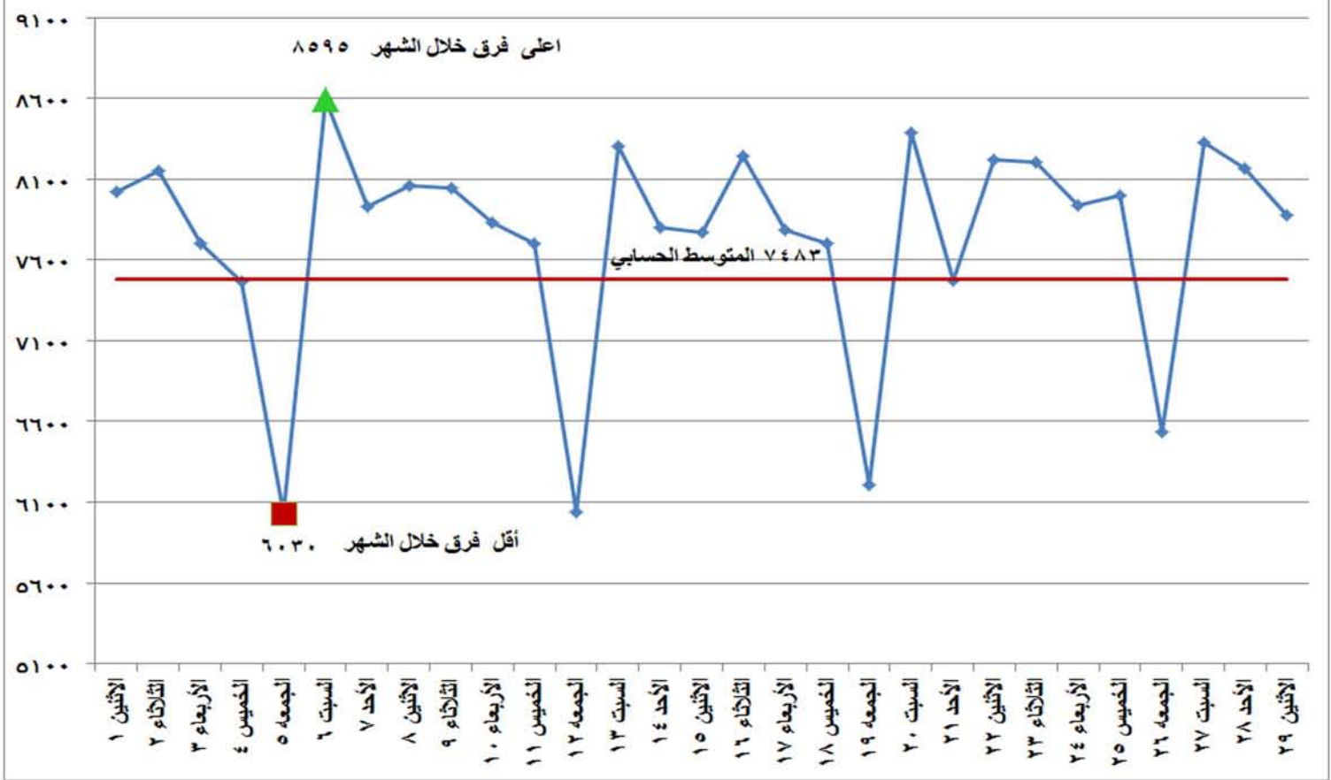
شكل (٣) الفرق بين أقصى وأدنى حمل خلال شهر فبراير ٢٠١٦
