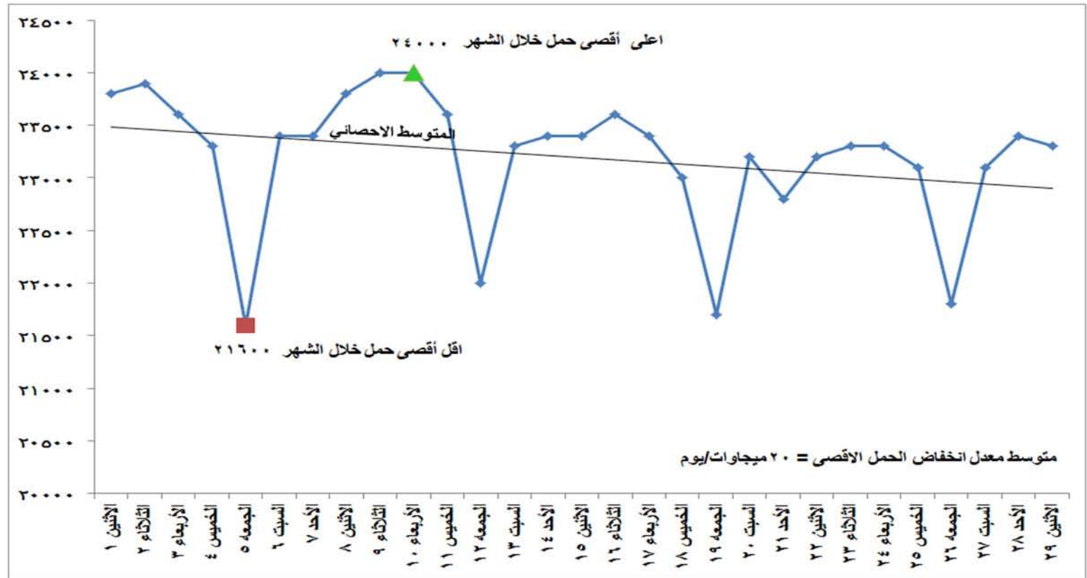
شكل (١) تطور الحمل الاقصى اليومي خلال شهر فبراير ٢٠١٦
