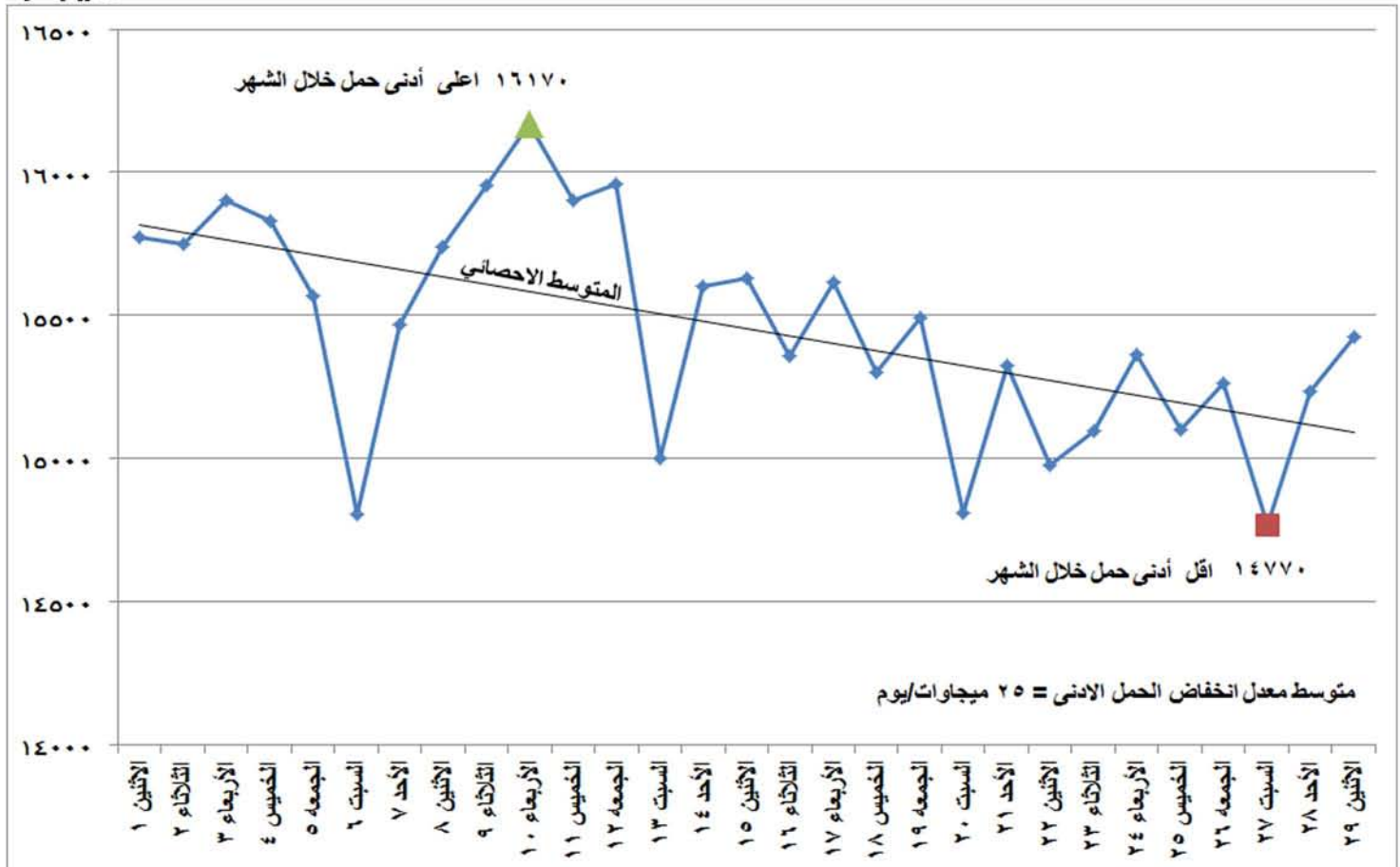
شكل (٢) تطور الحمل الادنى اليومي خلال شهر فبراير ٢٠١٦
