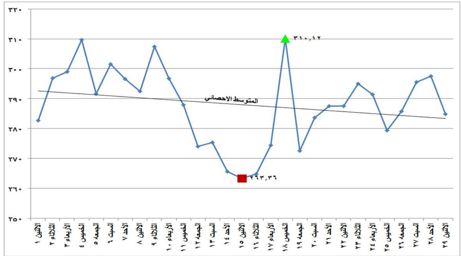
شكل (١٧) الطاقة الكهربائية المنتجة من الغاز الطبيعي خلال شهر فبراير ٢٠١٦
