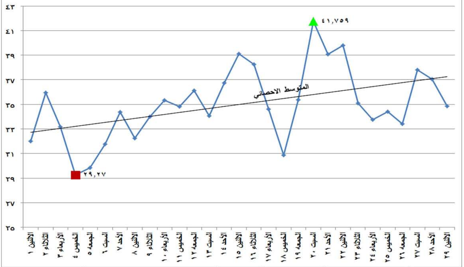
شكل (٢١) الطاقة الكهربائية المنتجة من المصادر غير الحرارية خلال شهر فبراير ٢٠١٦
