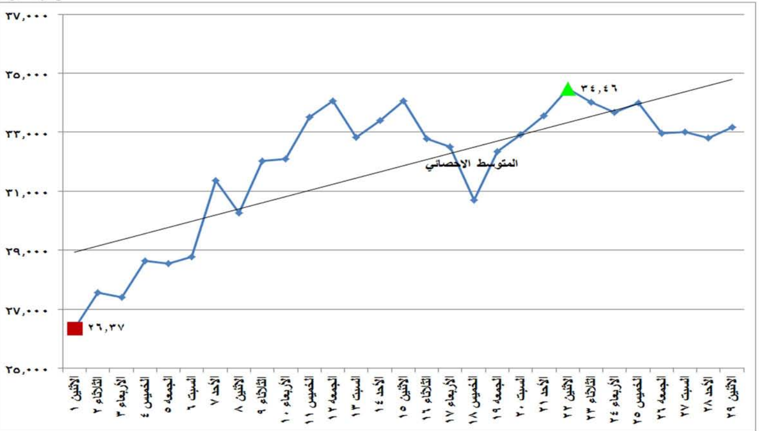
شكل (٢٣) الطاقة الكهربائية المنتجة من المصادر المائية خلال شهر فبراير ٢٠١٦
