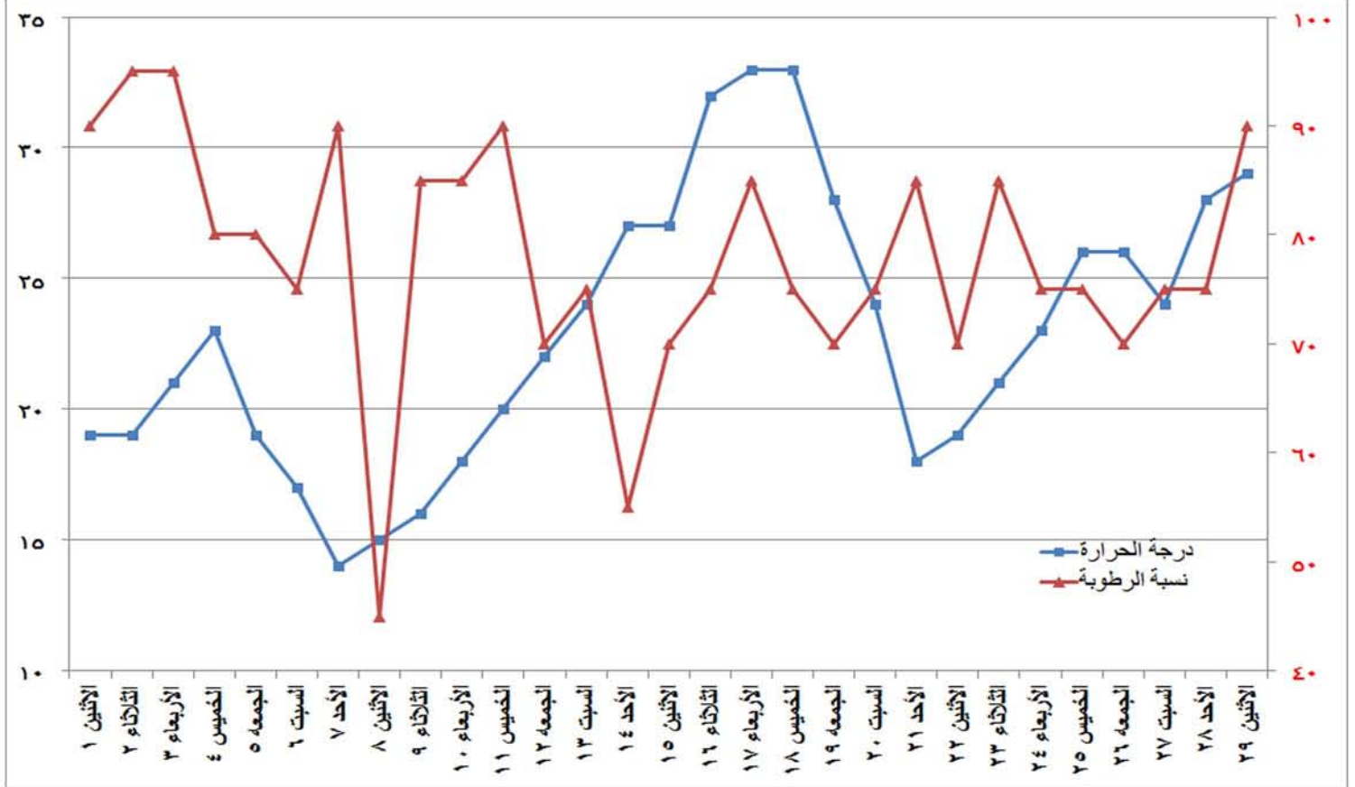
شكل (١١) التغيير في درجة الحرارة والرطوبة النسبية خلال شهر فبراير ٢٠١٦
