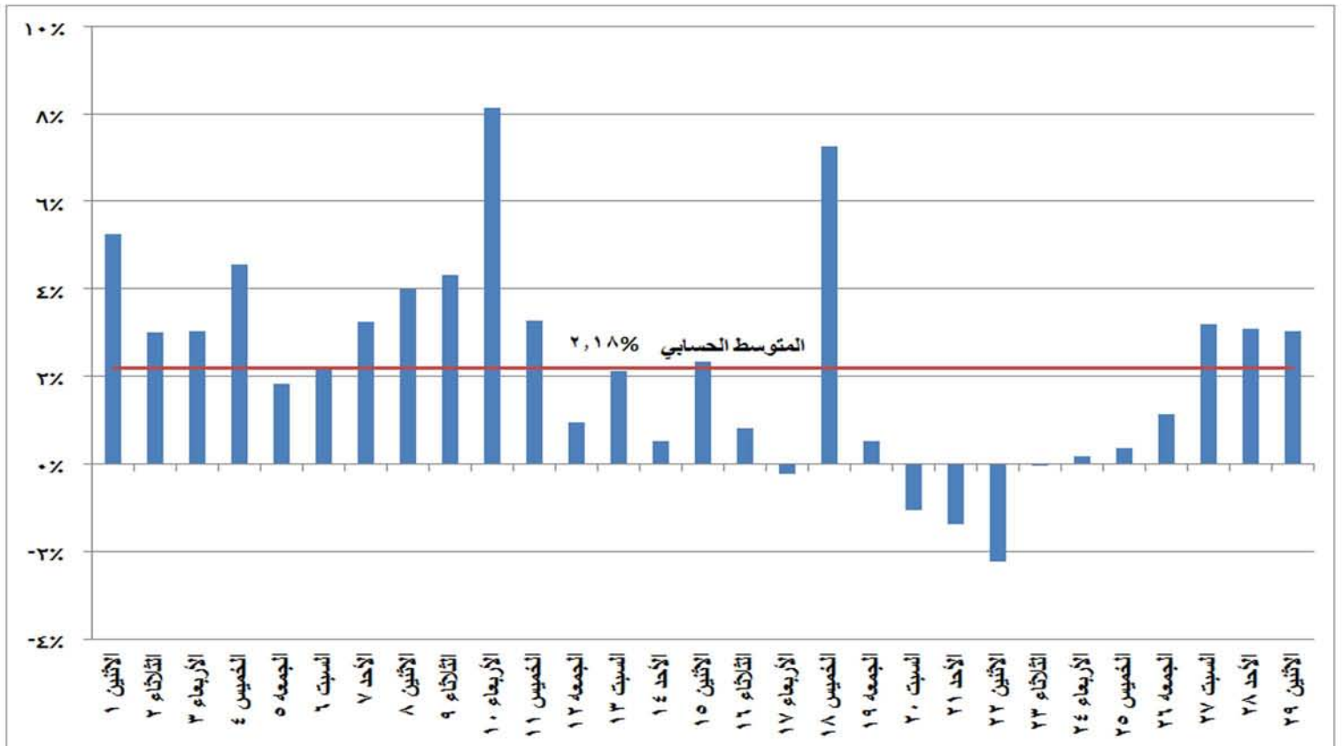
شكل (١٦) نسب التغير في الطاقة الكهربائية المنتجة خلال شهر فبراير ٢٠١٦ مقارنة بالشهر المماثل من العام السابق
