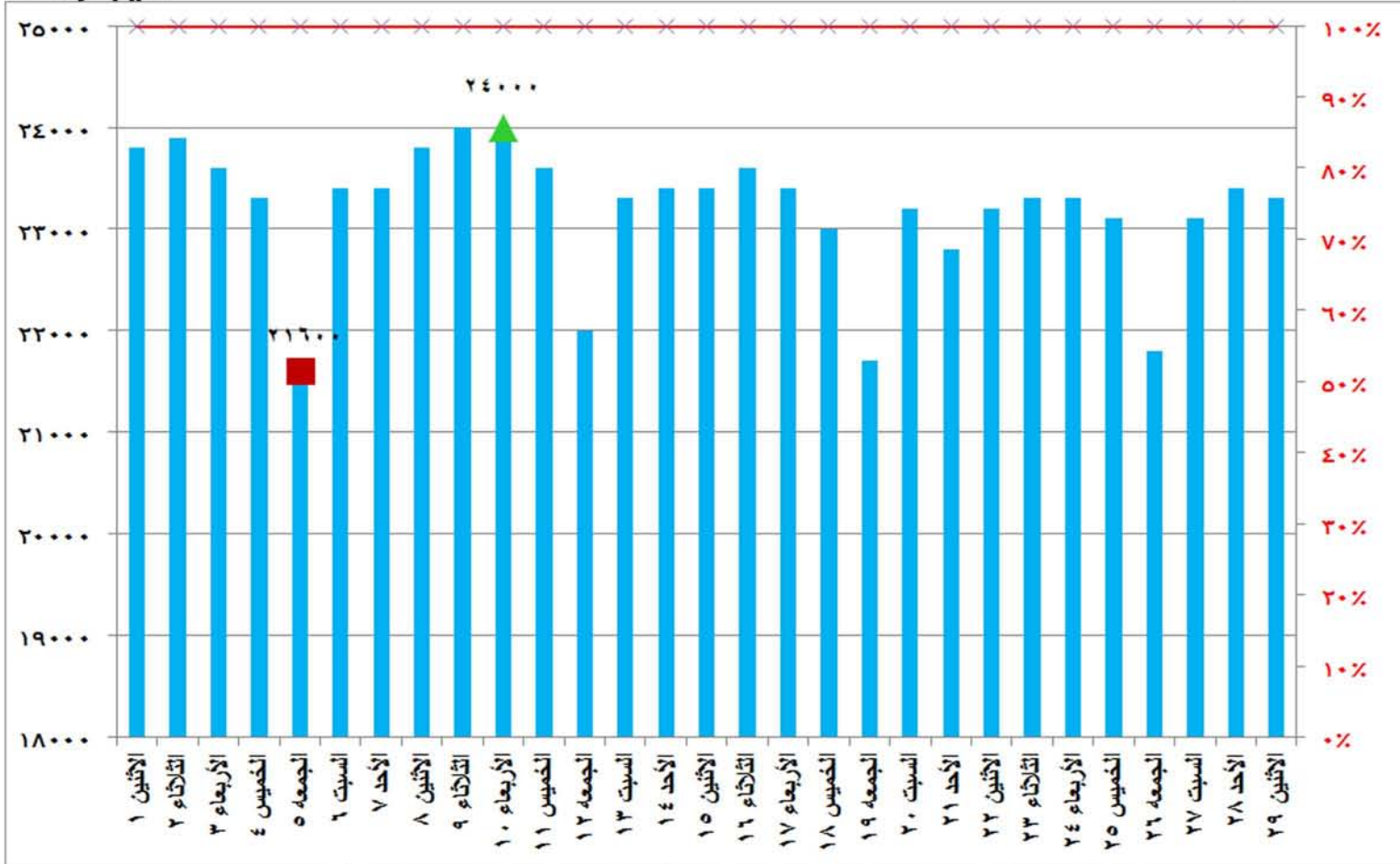
شكل (٥) قدرات الانتاج المتاحة ونسبتها للحمل الأقصى خلال شهر فبراير ٢٠١٦
